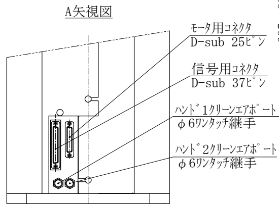
外部接続ハネ詳細図
