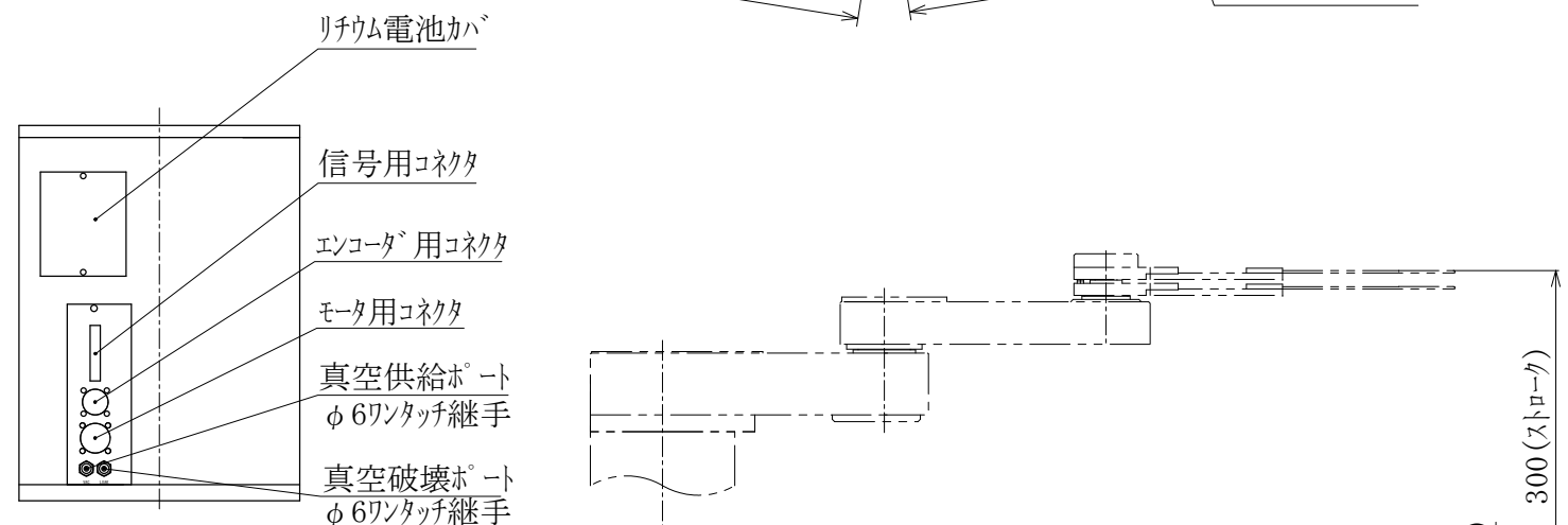
外部接続ポート詳細図
