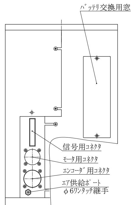
外部接続パネル詳細図
