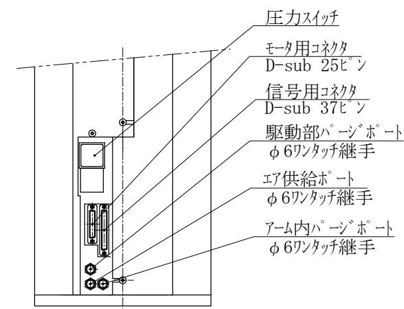
外部接続ハネ詳細図
