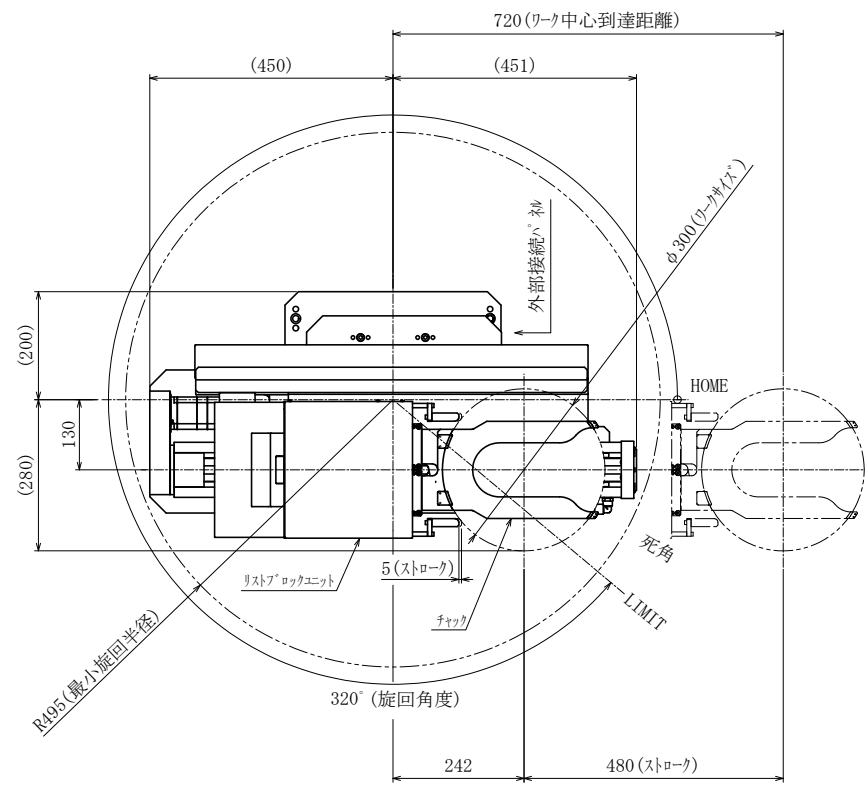
原点位置図
